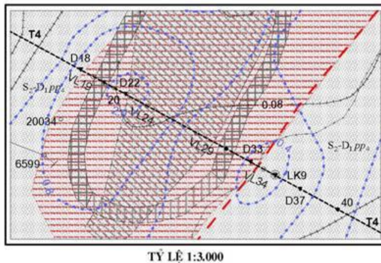
Hình 1. Sơ đồ địa chất và khoáng sản vùng Yên Thổ.
