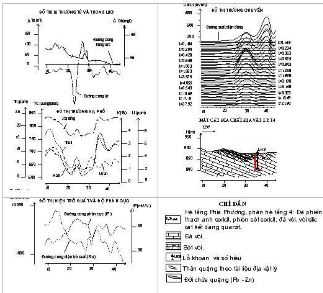
Hình 2. Mặt cắt địa vật lý địa chất tuyến 4 khu Yên Thố.
